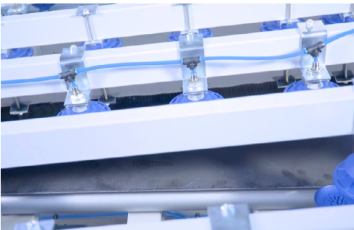
Stap 3 en 4: Glasplaten gecontroleerd uit elkaar trekken, platen in chemisch bad plaatsen om halfgeleiderlagen op te lossen, metaalfractionen (zoals Cd, Te) uit de oplossing terugwinnen
