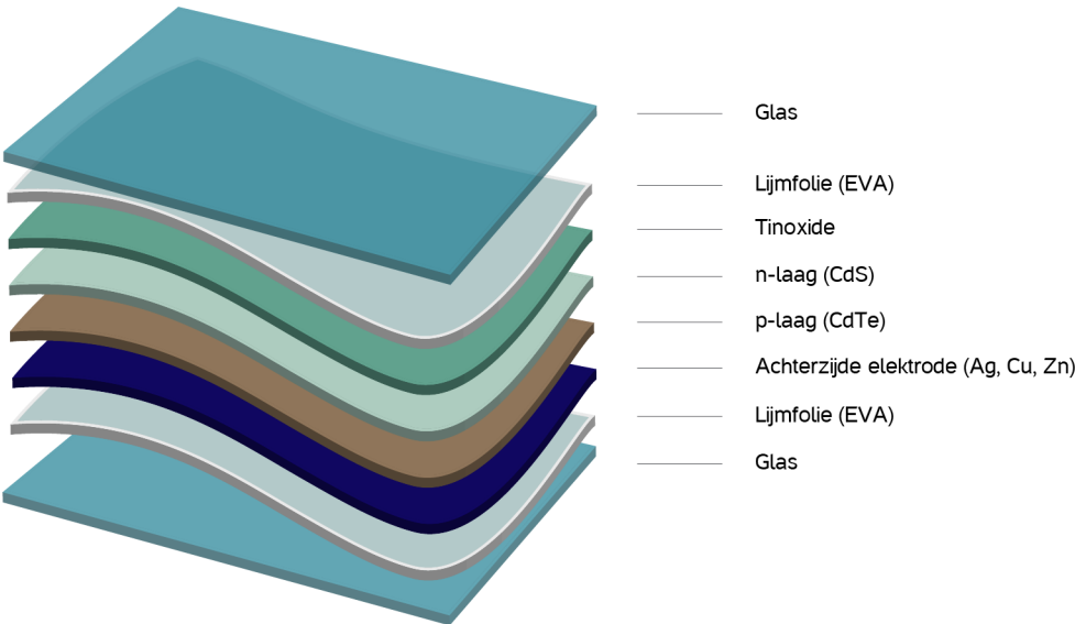
Dunne film (CdTe) Paneel
