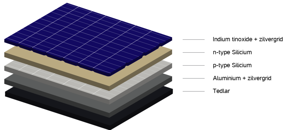
Si-paneel - opbouw van de cel
