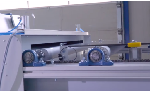
Stap 2: Paneel op rolband plaatsen en belichten in laserkamer, zodat hechting minder sterk wordt
